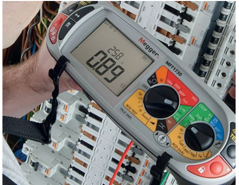
Instalaciones electricas
